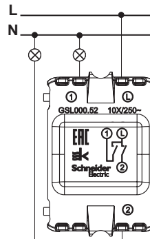
2-клавишный ВЫКЛЮЧАТЕЛЬ
